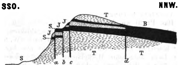
Fig. 2. Profil durch die Schichten von Gröf. B = Basalt; T = vulkanischer Tuff; J = Jökullhlaupsediment (Vulkanoglazial); S = Schliffflächen; a , b , c , d Verwerfungsspalten.
